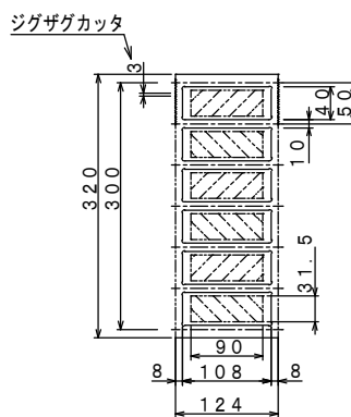
包装寸法 (2x6=12切)
