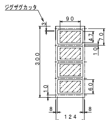
包装寸法 (2x4=8切)
